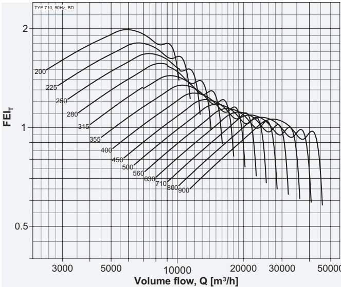
Model: TYE 710
